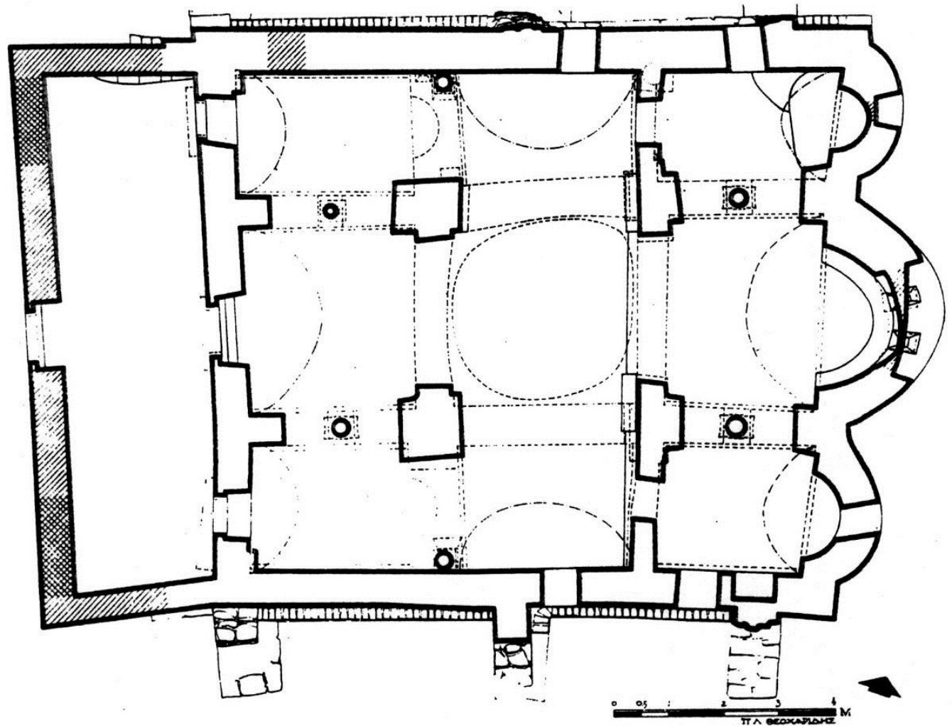
Πλησιοί Άρτας, "Άγιος Δημήτριος του «Κατσούρη», π. 800. (κάτοψη).
