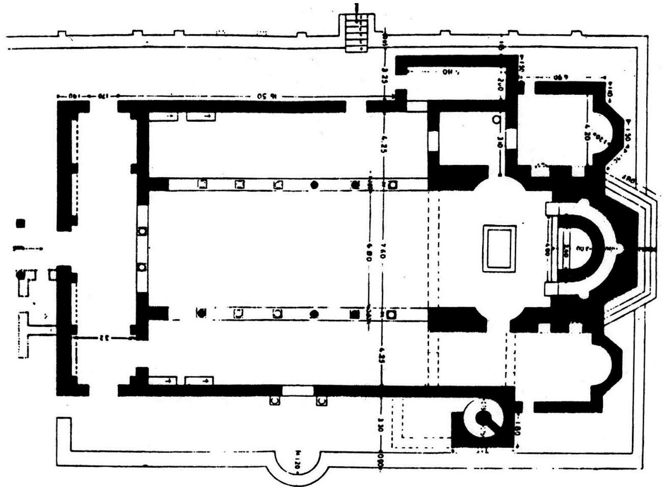
Σπάρτη, Βασιλική «όσιου Νίκωνος», 7ος αι. (κάτοψη).
