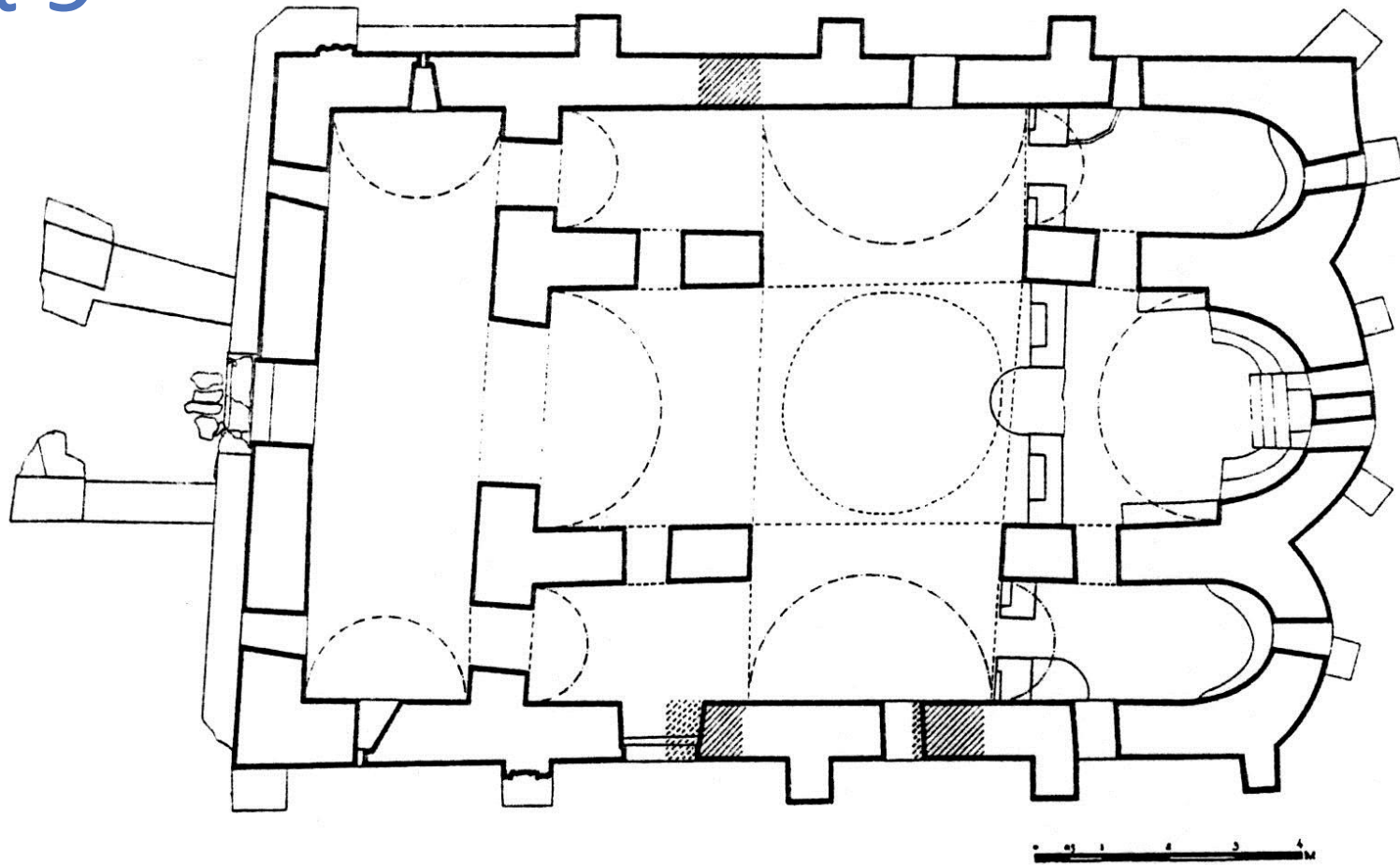
Ευρυτανία, Ἐπισκοπή, π. 800 (κάτοψη).
