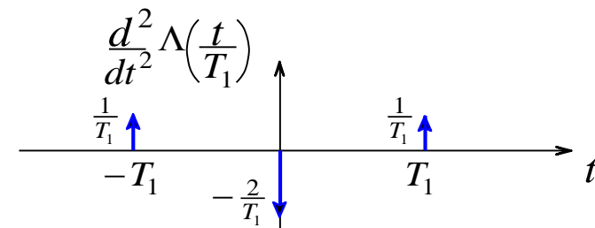
Η δεύτερη παράγωγος του τριγωνικού παλμού διάρκειας 2T_1 .
