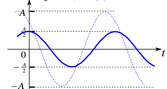
Η έξοδος του συστήματος όταν f_0 = 1500 Hz.
