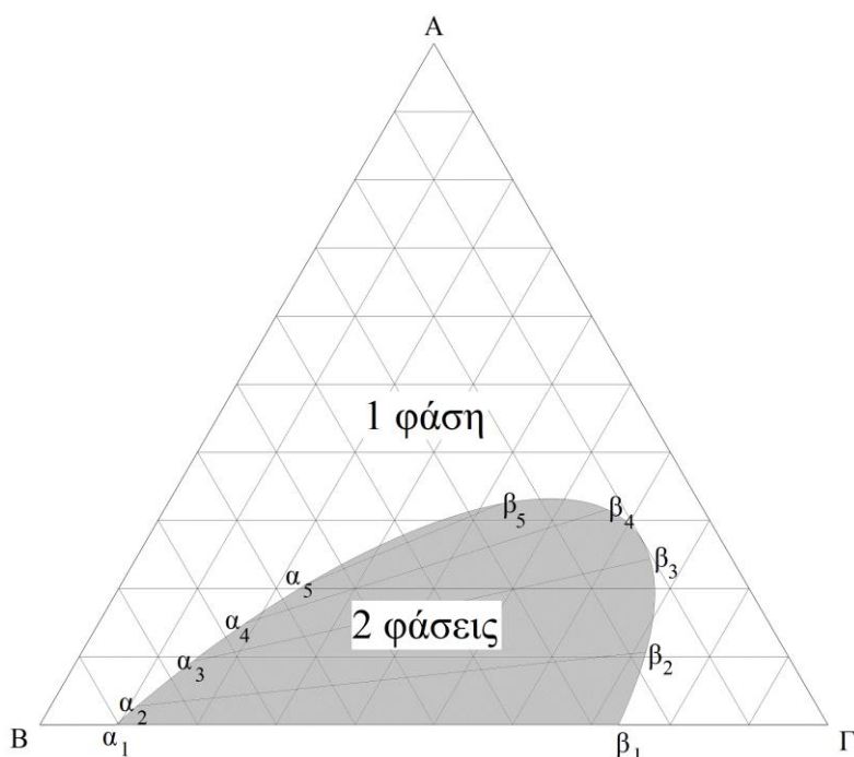
Σχήμα 2: Τριγωνικό διάγραμμα φάσεων συστήματος τριών συστατικών
